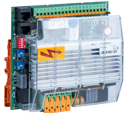
Bremsgerät VB S LP [60A]
