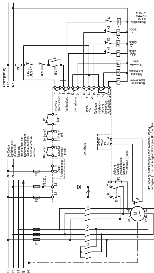
17.4 Standard Anschlussplan mit allen Optionen VB ...-100...600
