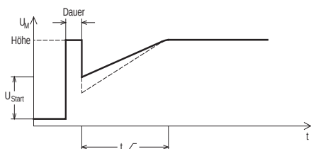
Diagramm für Start mit Spannungsrampe und Boost
