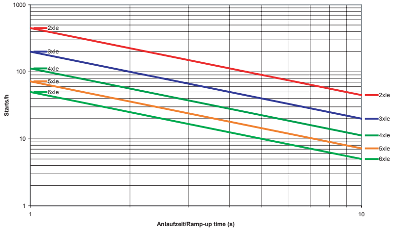
VersiStart II 400-25
