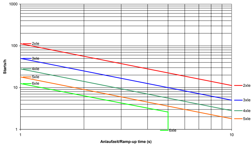
VersiStart II 400-45
