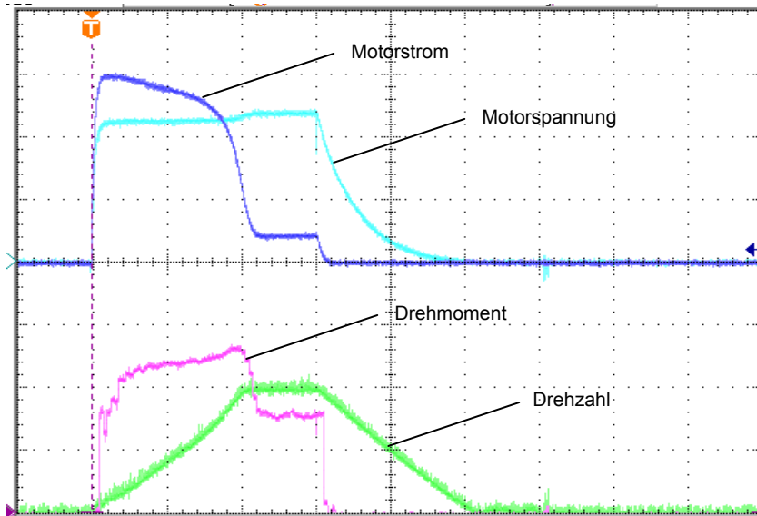
Anlauf eines Drehstromsynchronmotors mit Nennlast direkt am Netz
