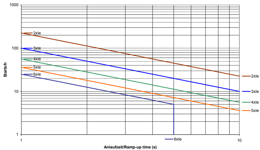
VersiStart II 400-75
