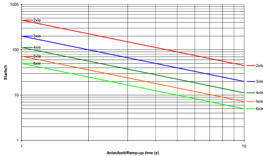
VersiStart II 400-25
