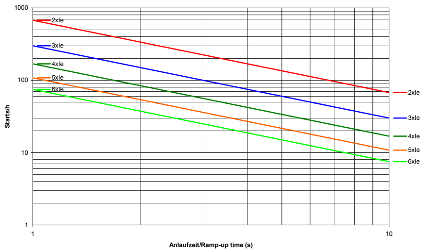
VersiStart II 400-25
