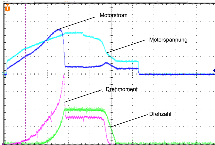
Anlauf eines Drehstromsynchronmotors mit einem Sanftanlaufgerät und Nennlast
