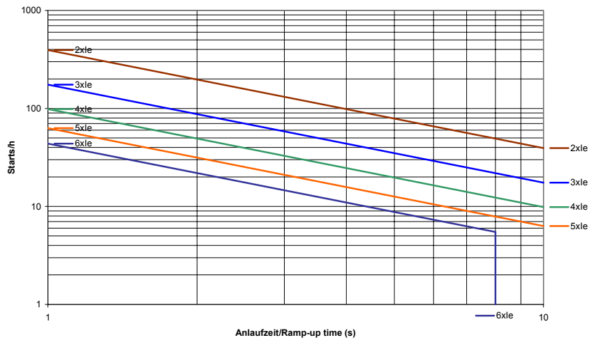
VersiStart II 400-50
