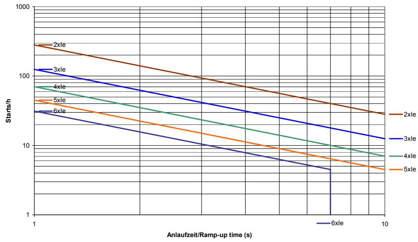
VersiStart II 400-65
